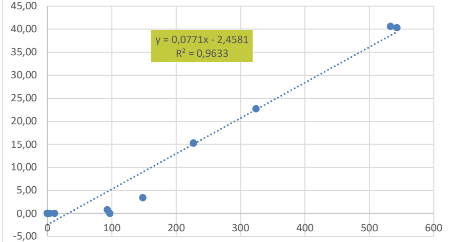
Doğalgaz Tüketimine Göre Regresyon Analizi
